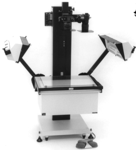
型式：FD (ステージ電動昇降式) 光源：蛍光灯 ステージサイズ：612×460 mm
